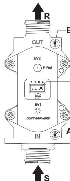
рис. 18 - Газовый клапан
