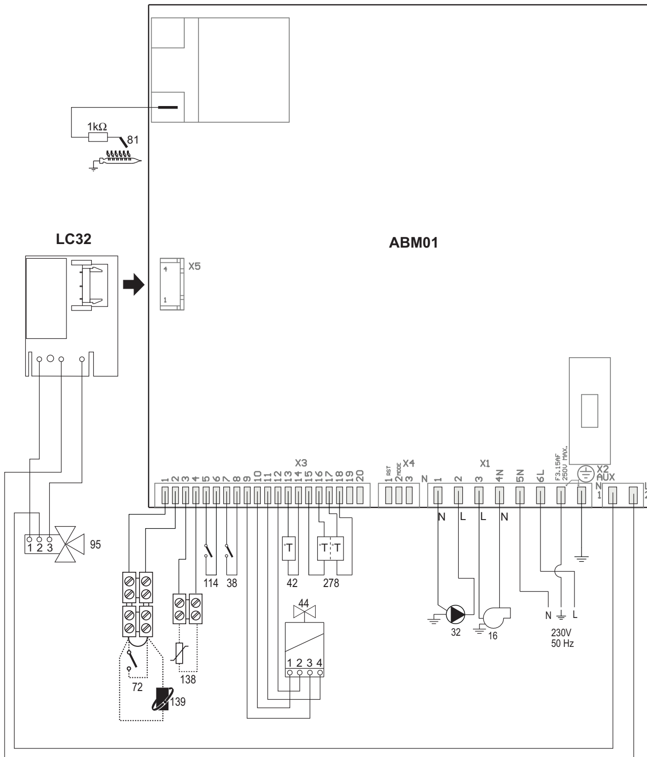
рис. 24 - Электрическая система
