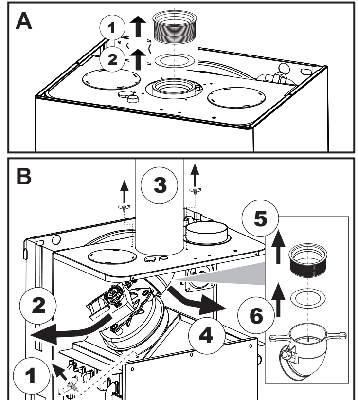
А Замена диафрагмы, когда котел еще не установлен
